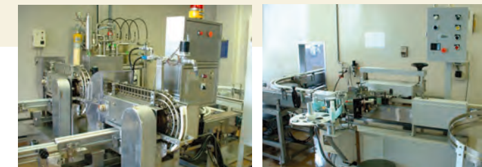
機械名：内用液剤充填ライン 機械メーカー：シバヤ精機株式会社 充填量：10ml、30ml 運転速度：10ml～50本/分、30ml～32本/分 接液部材質：SUS316製 硬質クロムメッキ付 機器構成：リンサー→10ml用 森本鉄工所 MR2050型 →30ml用 森本鉄工所 MR2080型 フィラ 造谷工業 RF09-09TV型 パーツフィード 造谷工業 PKF5000型 マルチキョッパ 造谷工業 PCM1000型 タックラベラ タカラ ALB-100型 ボトルコンベヤ 造谷工業 Z7700B型 自動除菌装置 達生テック T-1030型
